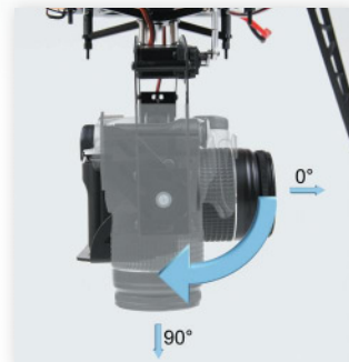
Schwenkbare Kamerahalterung
